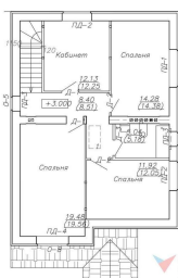
План на отм. +3.000.
