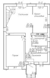
План на отм. 0.000, -0.200.
